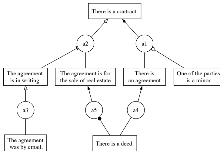
Fig. 1. Argument Graph
